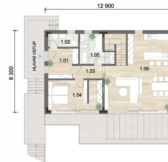
PŮDORYS 1NP
