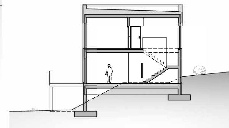
ŘEZ PŘÍČNÝ
